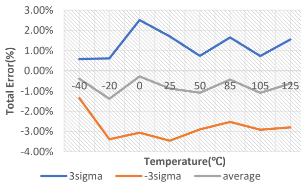
图 6: 线性输出 vs. IP 误差图
