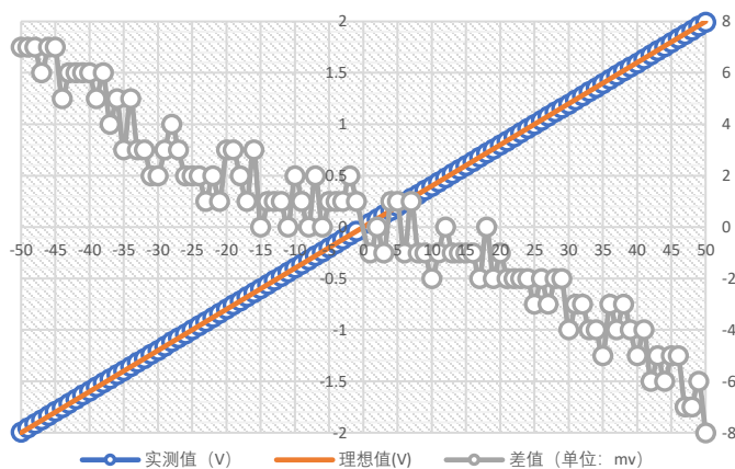
图 6: 线性输出 vs. IP 误差图
