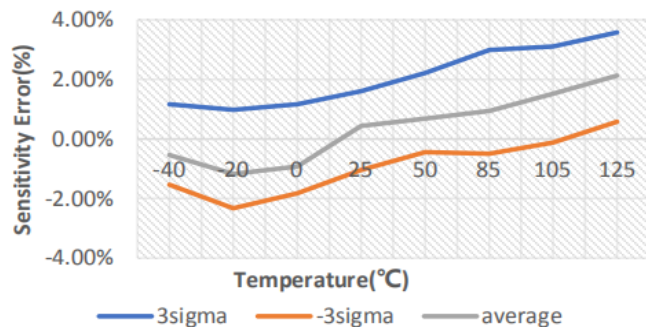
图 7：总精度误差温漂
