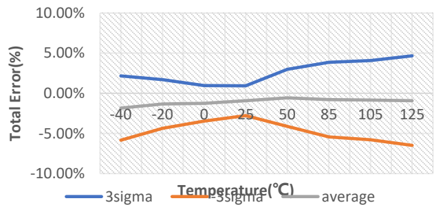
图 7：总精度误差温漂
