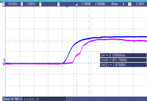
图 3: 响应延迟时间图
