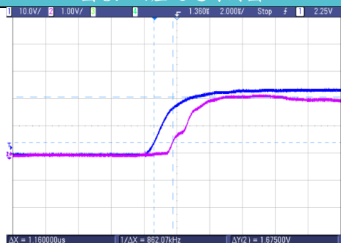
图 5: sinwave 瞬态响应图
