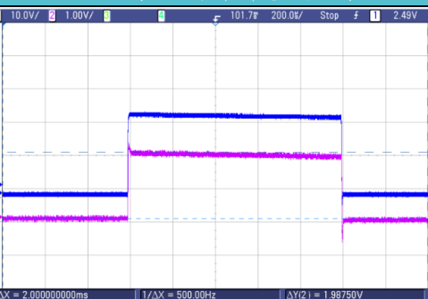
图 6: 脉冲瞬态响应图
