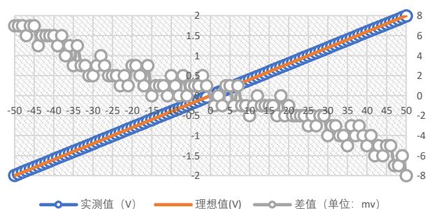
图 8：线性输出 vs.IP 误差图
