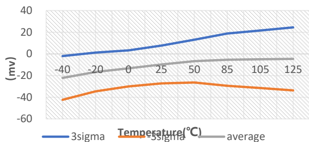
图 3：零点输出电压温漂
