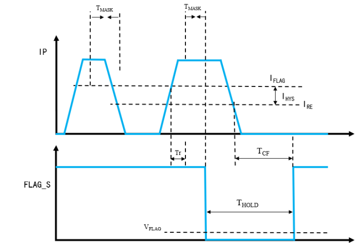
图 3: Tmsk 功能启用时 FLAG_S 时序图
