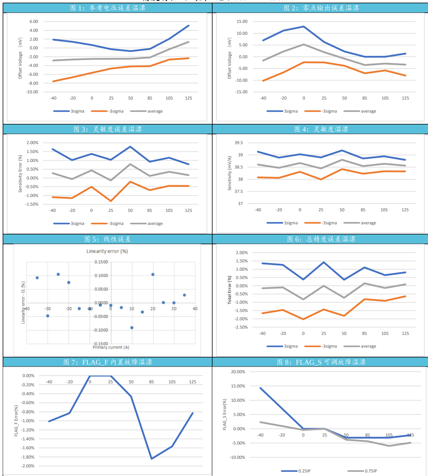
精度特性曲线图 (基于 SC824BFT-35G5)
