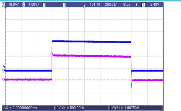
图 6: 脉冲瞬态响应图
